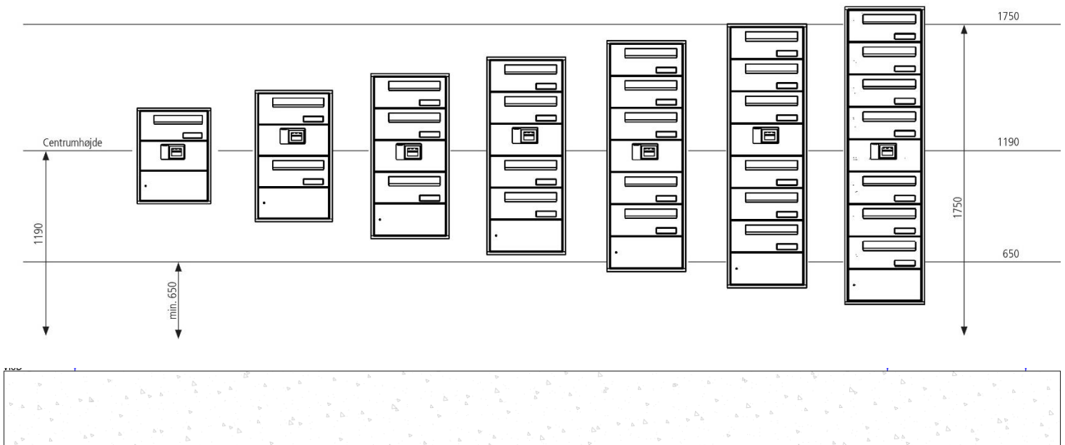
Illustration af syv postkasseanlæg, hvor de er placeret på væggen, således at deres centrumlinje er 1190 mm over gulvet.
